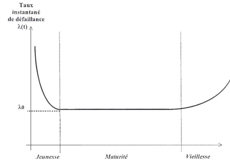
Illustration 21 : évolution du taux de défaillance en fonction du temps
