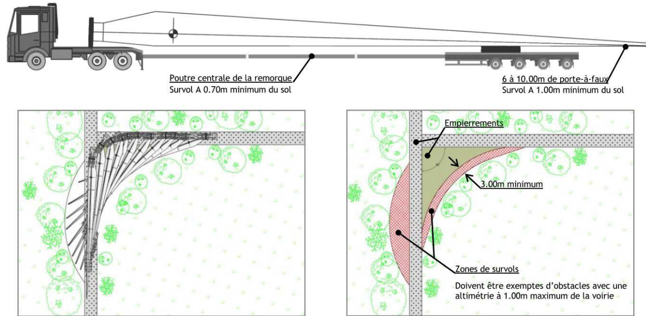
Illustration 13 : porte à faux des pales et zones de survols lors du transport (source : Vestas)
