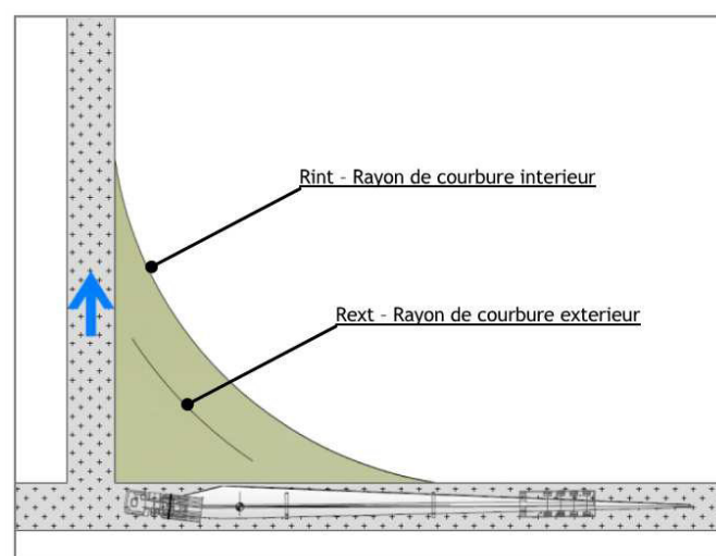
Illustration 17 : aménagement des virages
