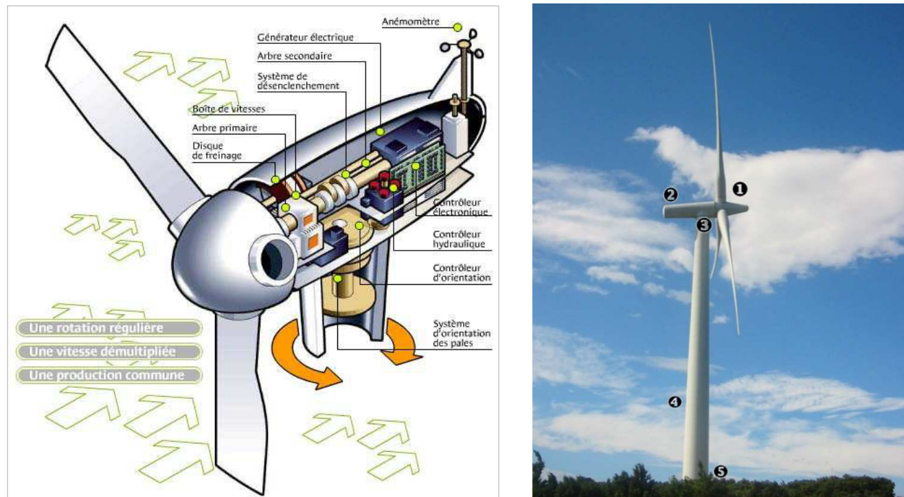
Illustration 5 : l'éolienne
