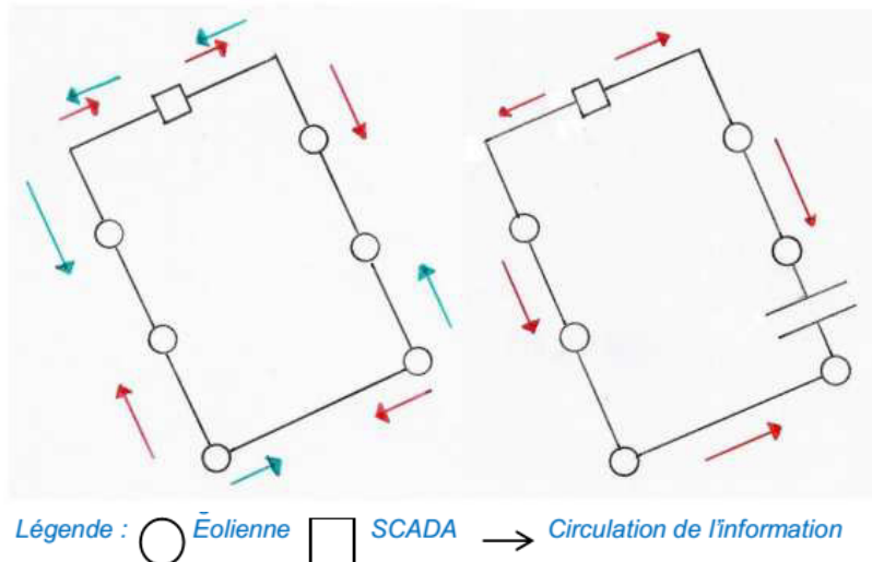
Illustration 20 : système en anneau garantissant une communication continue des éoliennes
