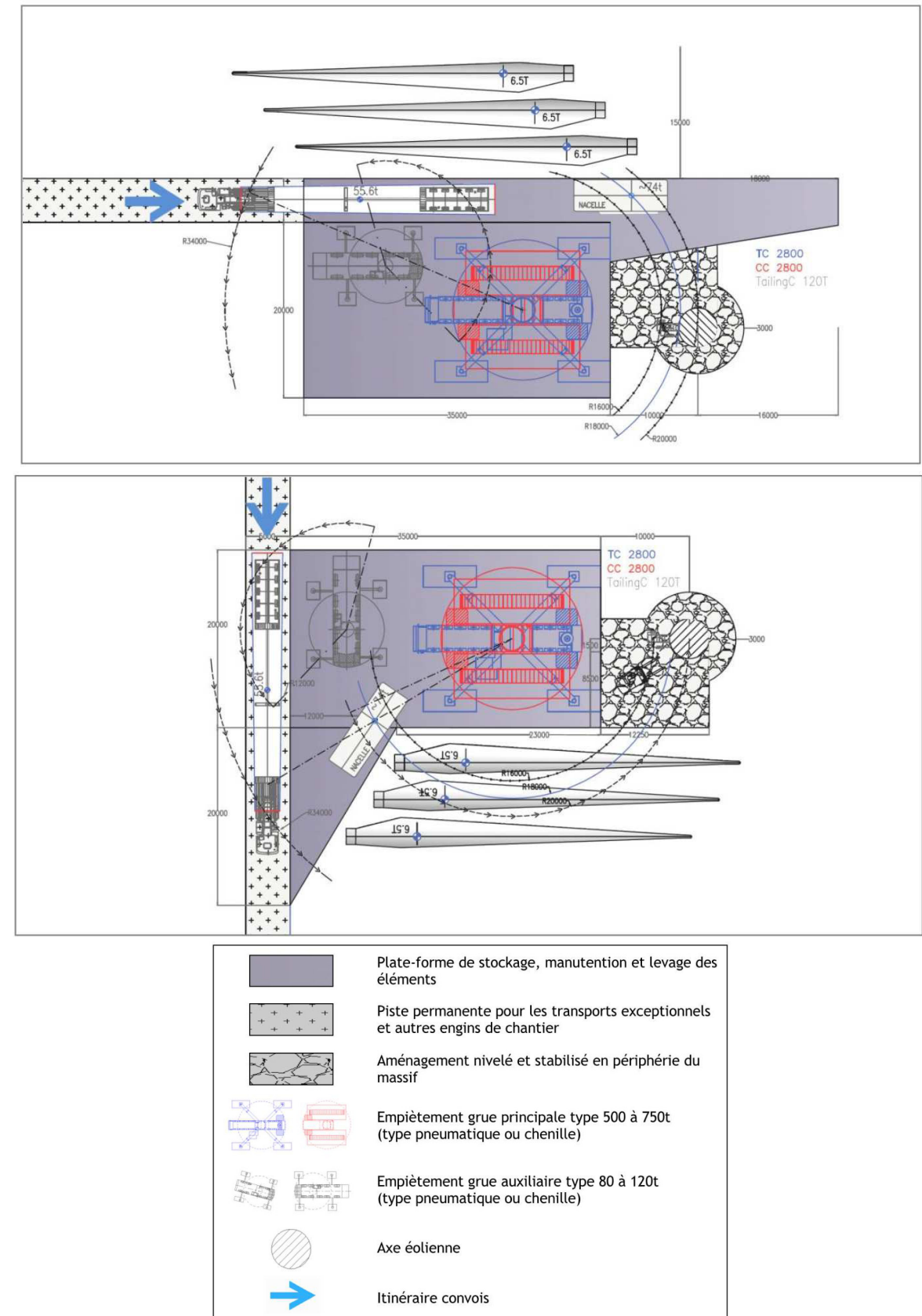
Illustration 18 : principe d'organisation d'une plateforme (exemples en bout de piste et perpendiculaire à la piste - source : Vestas)
