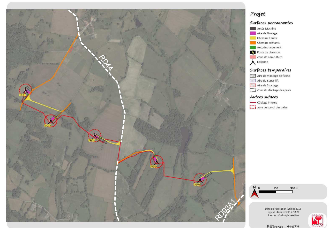
Illustration 7 : accès aux différentes zones d'implantation des éoliennes depuis les départementales
