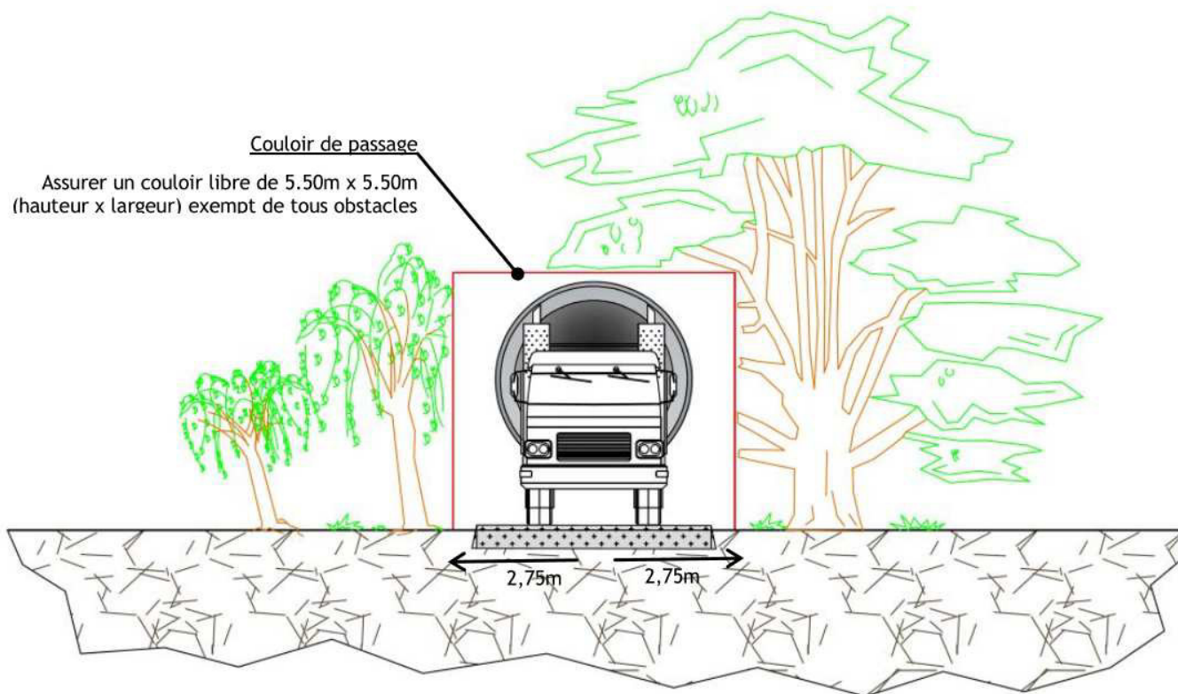
Illustration 14 : couloir de passage utile (source : Vestas)
