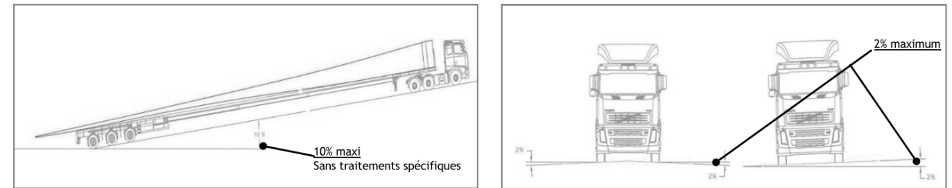
Illustration 15 : pentes longitudinales et transversales pour le transport
