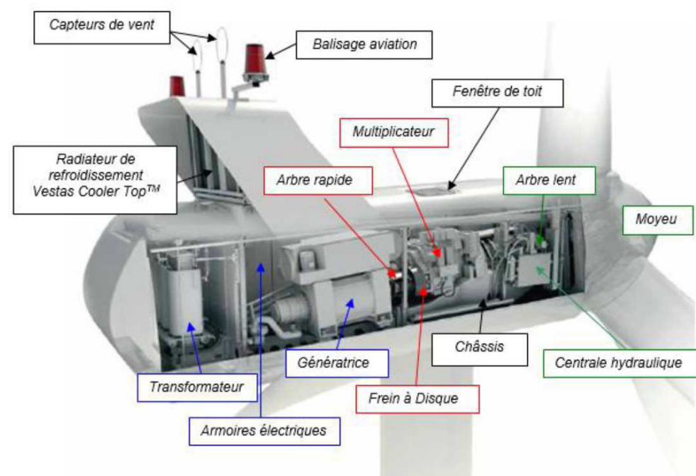
Illustration 9 : Ecorché simplifié de l'intérieur de la nacelle VESTAS V110 (source : documentation VESTAS, 2016)
